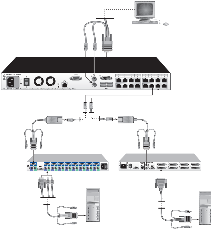
Figura 2-13. Configuración de conexión en cascada del conmutador de consola remota con conmutadores de consola existentes
